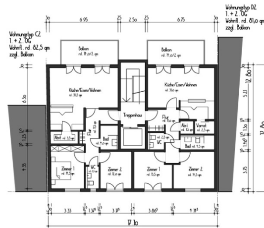
1. + 2. Obergeschoss
